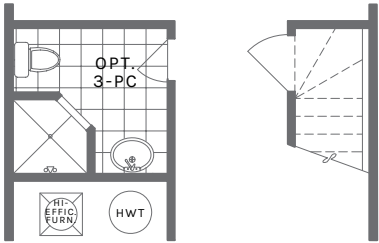
OPTIONAL 3-PC BATH PLAN
