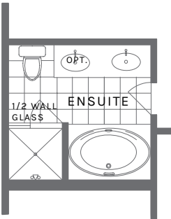
OPTIONAL ENSUITE PLAN W/ TUB
