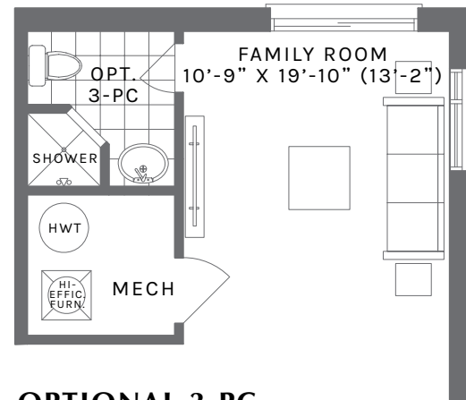
OPTIONAL 3-PC BATH PLAN
