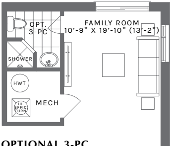
OPTIONAL 3-PC BATH PLAN
